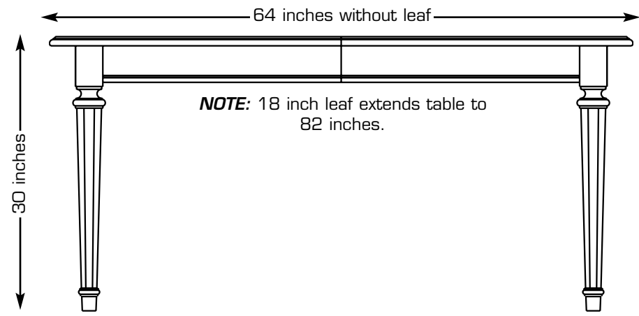
920-760 LEG TABLE
